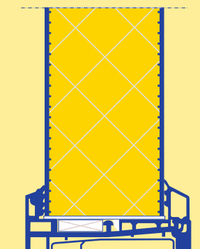
montage in kunststof en aluminium kozijn
