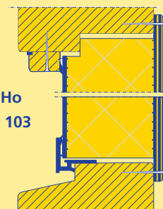
Houten kozijnen
