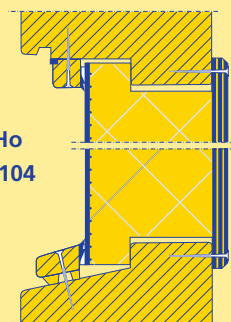
Houten kozijnen
