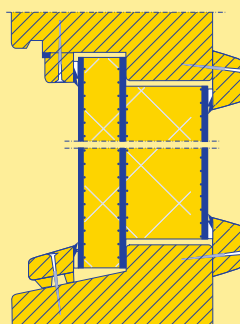
Houten kozijnen
